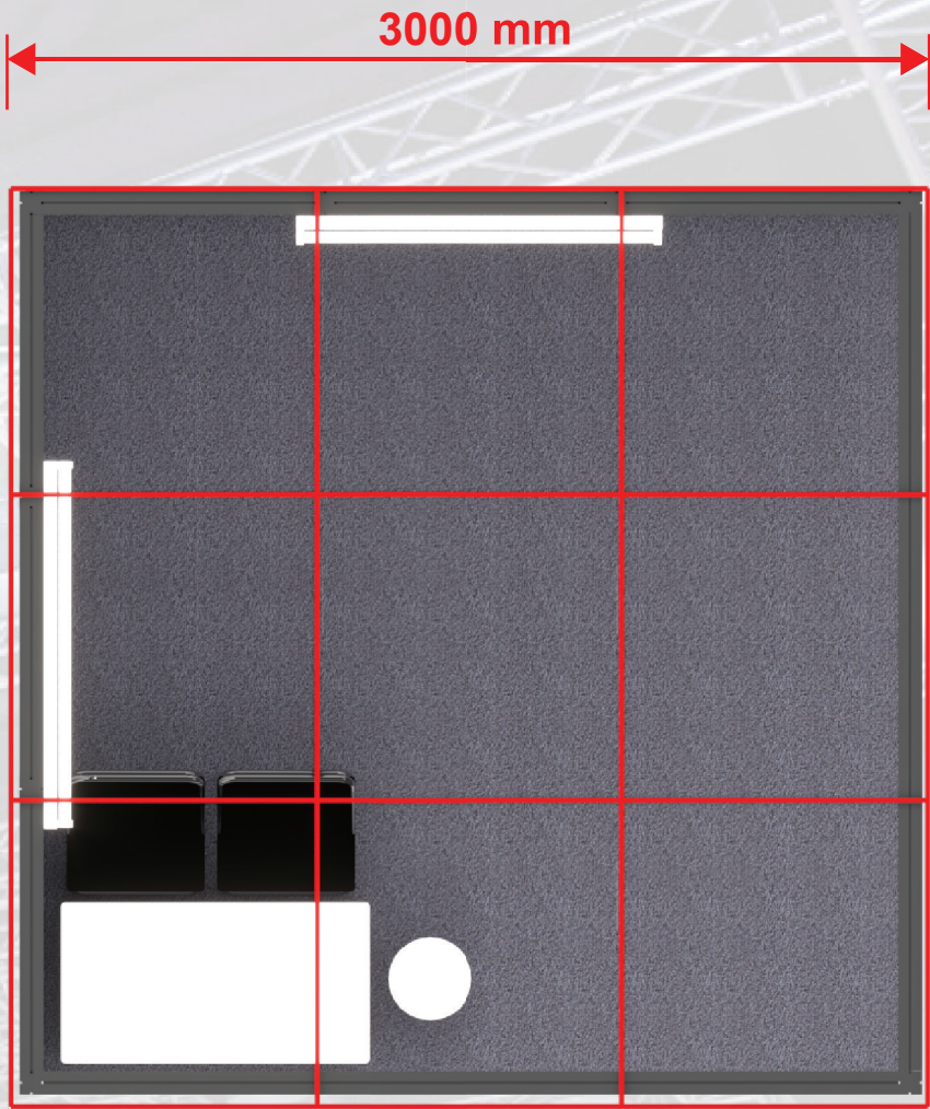
TOP ELEVATION
