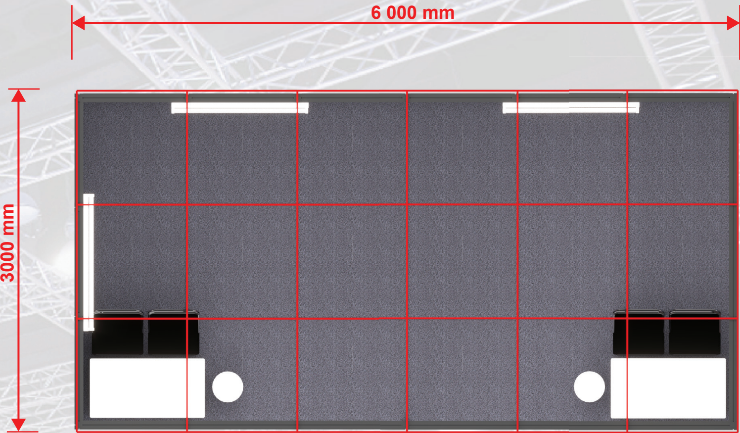
TOP ELEVATION
